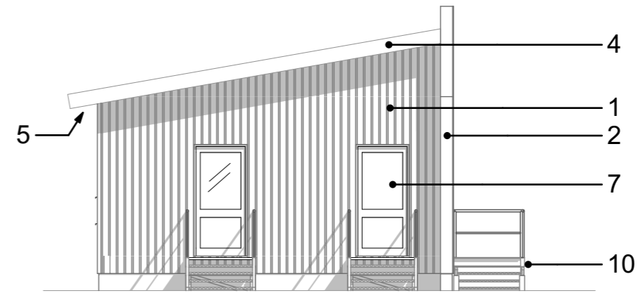
Julkisivu LÄNTEEN
