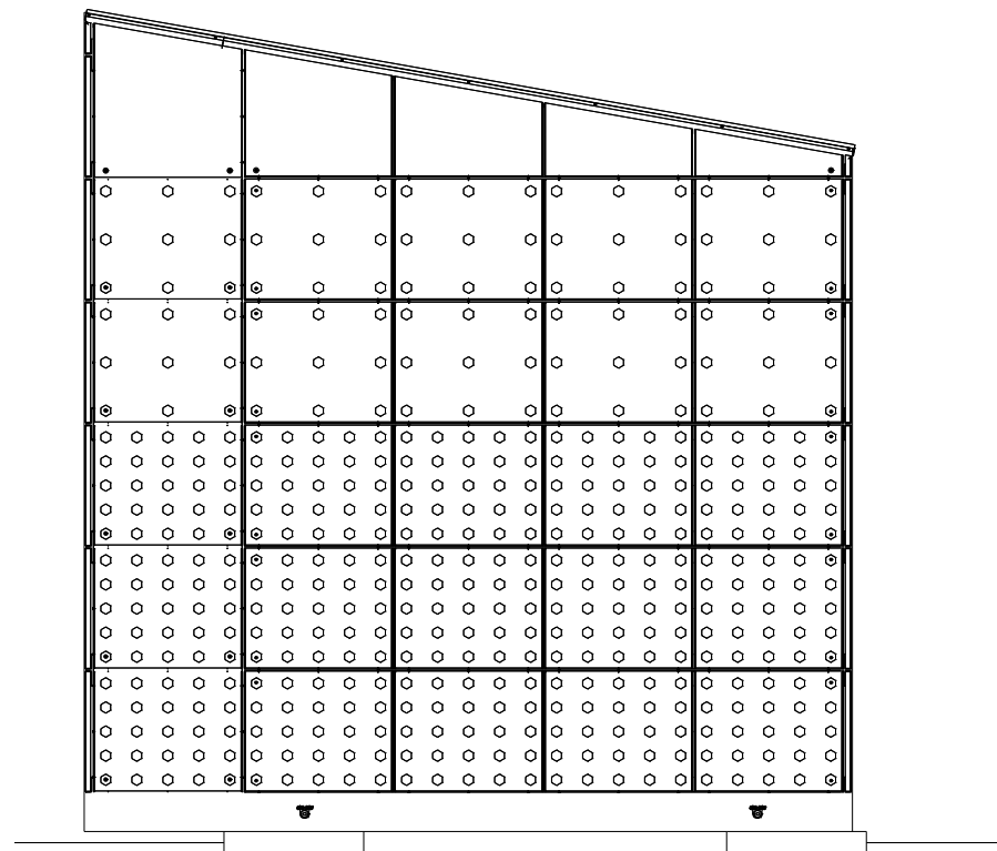
JULKISIVU, SIVU 1 1:30
