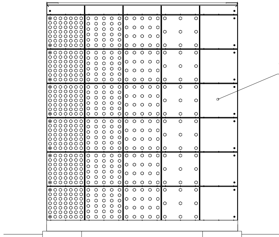
JULKISIVU, TAKASEINA 1:30
