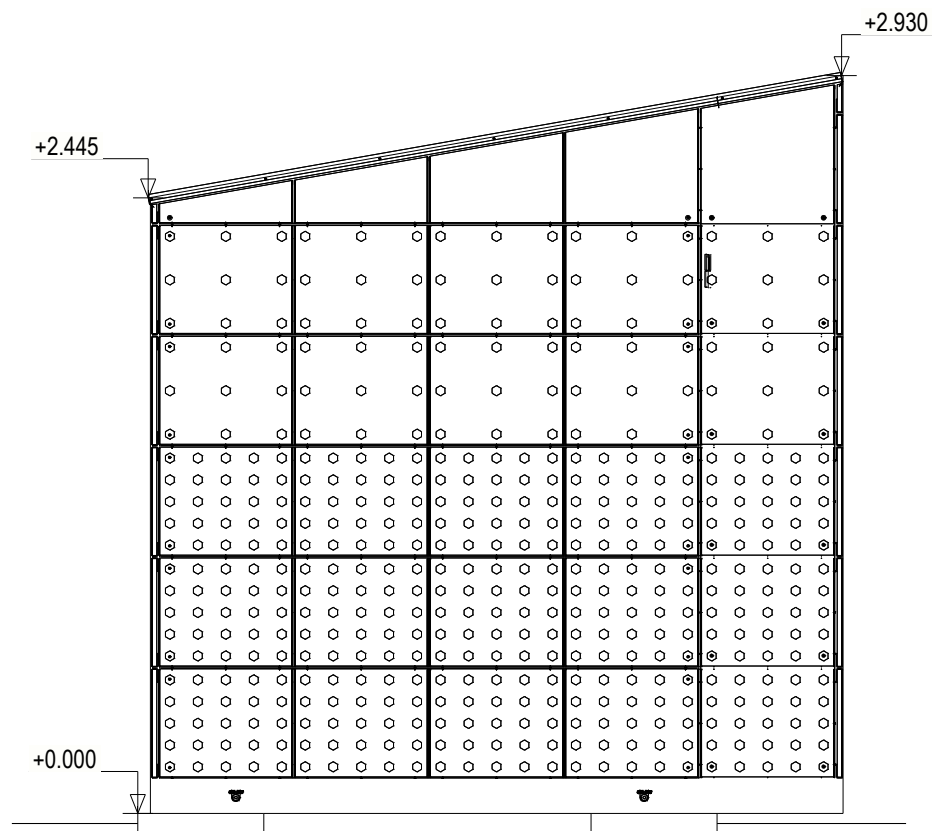
JULKISIVU, SIVU 2 1:30
