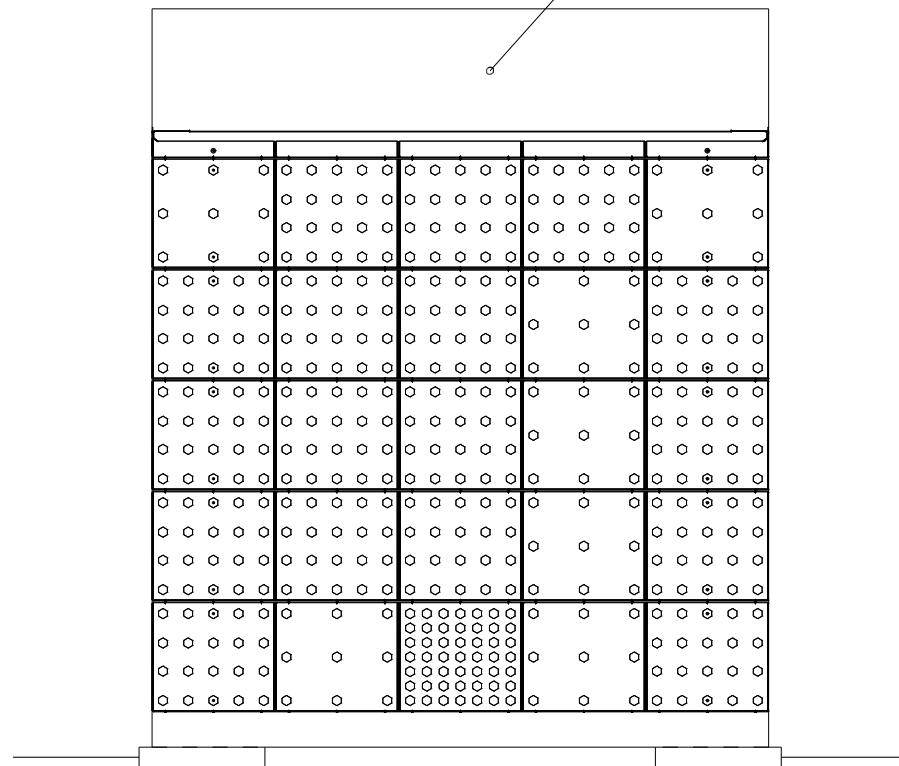
JULKISIVU, ETUSEINA 1:30
